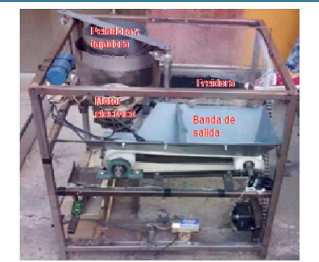
Fig. 8. Prototipo final de la peladora y tajadora de papa.
