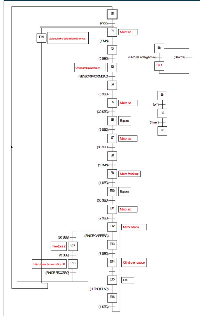
Fig. 5. Algoritmo de control de la máquina
