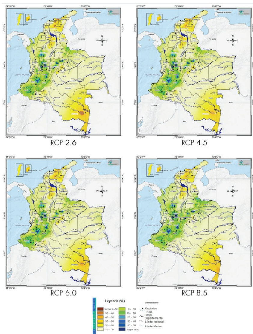
Figura 2. Cambio porcentual (%) de la precipitación en el periodo 2011-2040 frente al periodo 1976-2005 para Colombia según los RCP IDEAM (2015).
